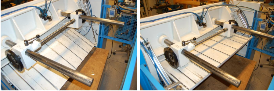
Bild 2: tv bordet nere, th bordet uppe.
