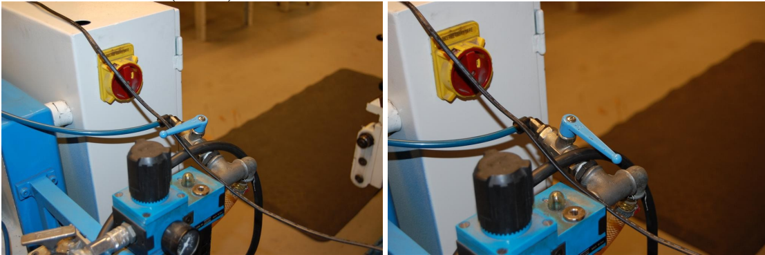
Bild 3: tv kranen avstängd, th kranen öppen (driftläge)
